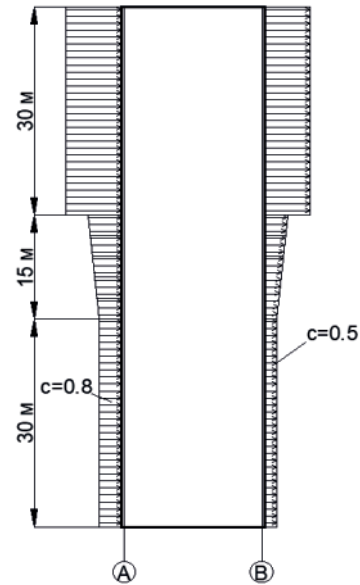
Рис. 2. Схема распределения ветровой нагрузки.
